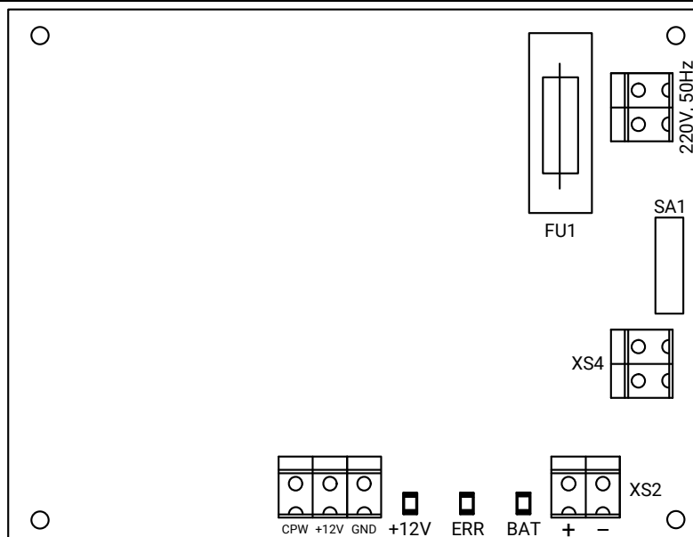
Рисунок 1. Плата прибора
